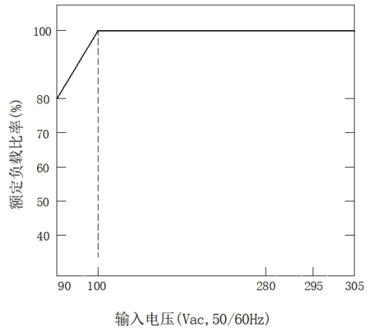
■ 输入电压与负载降额曲线
