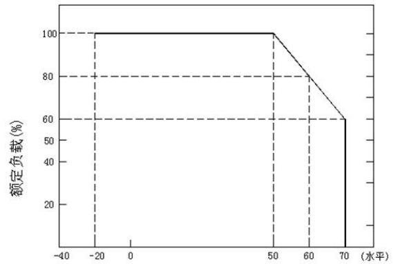
■ 环境温度VS额定功率降额曲线
